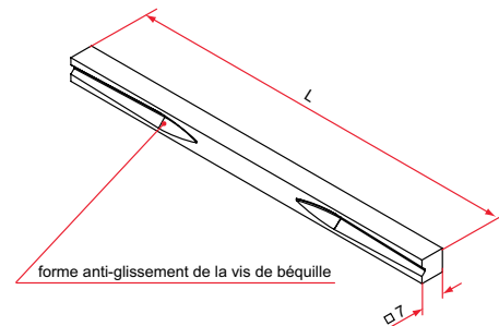
Rainure autobloquante
