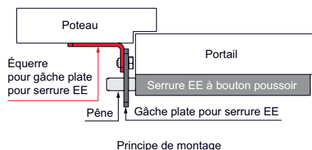
Principe de montage
