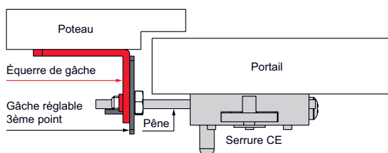
Principe de montage
