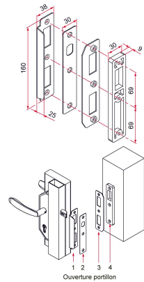
Rep 1 - Gâche butée Rep 2 - Têtière plate Rep 3 - Gâche plate Rep 4 - Cale d'épaisseur
