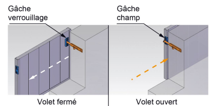
Principe de montage : montage en tableau à gauche ou à droite
